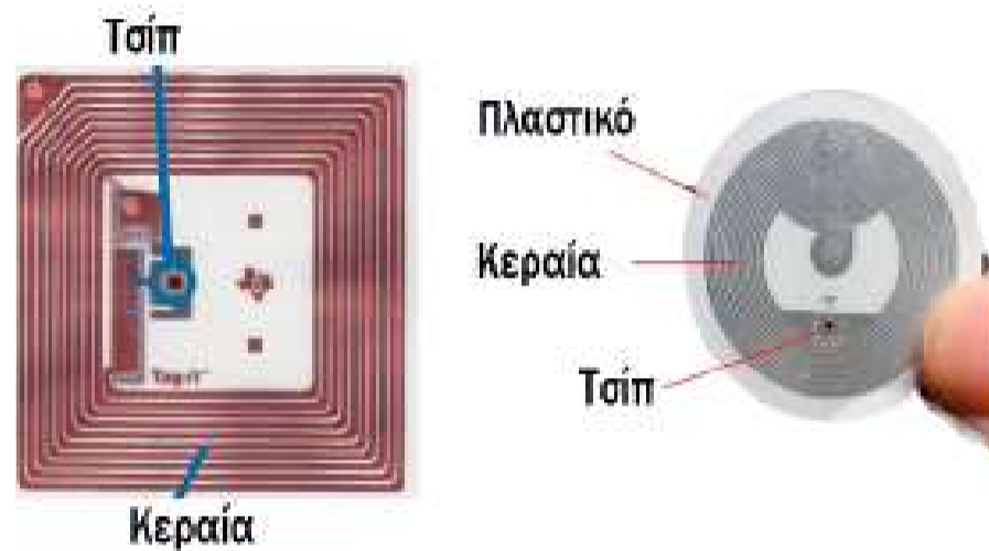
Πίνακας 2. NFC διάταξη: Η κεραία και το τσίπ (μπορεί να είναι ορθογωνίου ή στρογγυλού σχήματος) - Σημείωση: Και το RFID τσίπ είναι σχεδόν το ίδιο οπτικά
