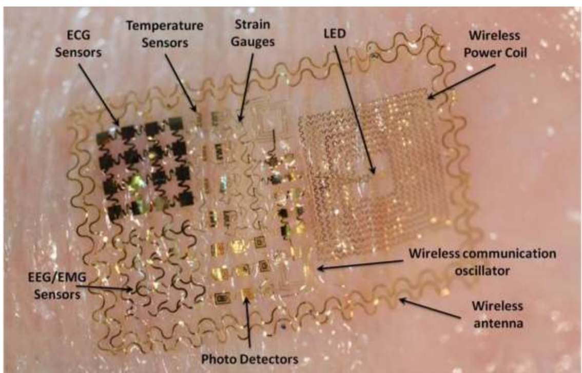
Πίνακας 8. Εὐκαμπτα ἐπιφανειακὰ “ἐμφυτεύματα” (σὰν τατουάζ)
